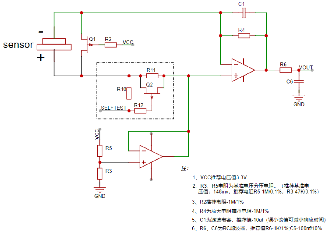
图 21 传感器自诊断电路示意图
