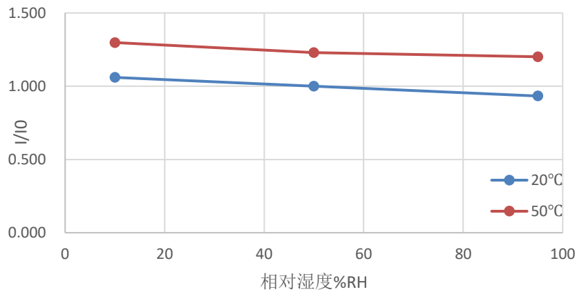
图 16 湿度影响
