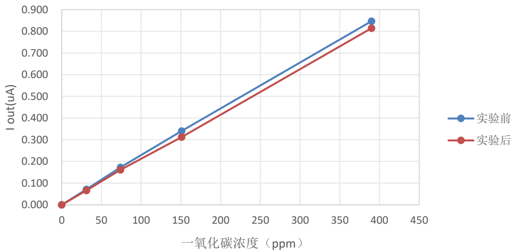
图 14 误报警测试
